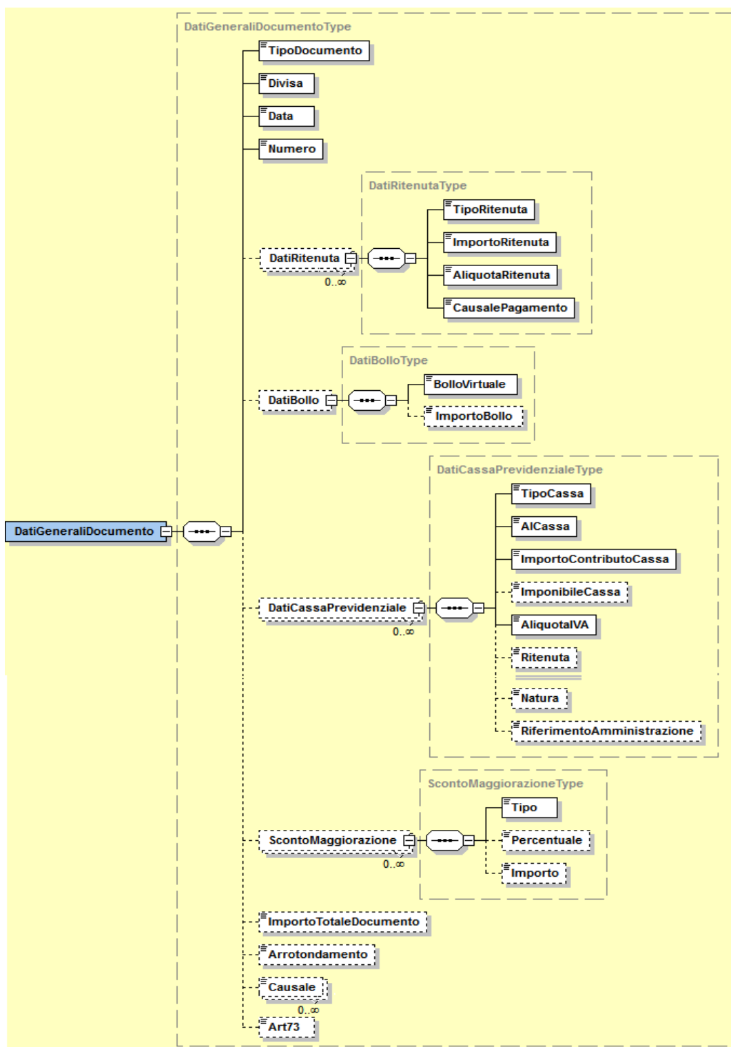
Figura 19: Elemento DatiGeneraliDocumento
