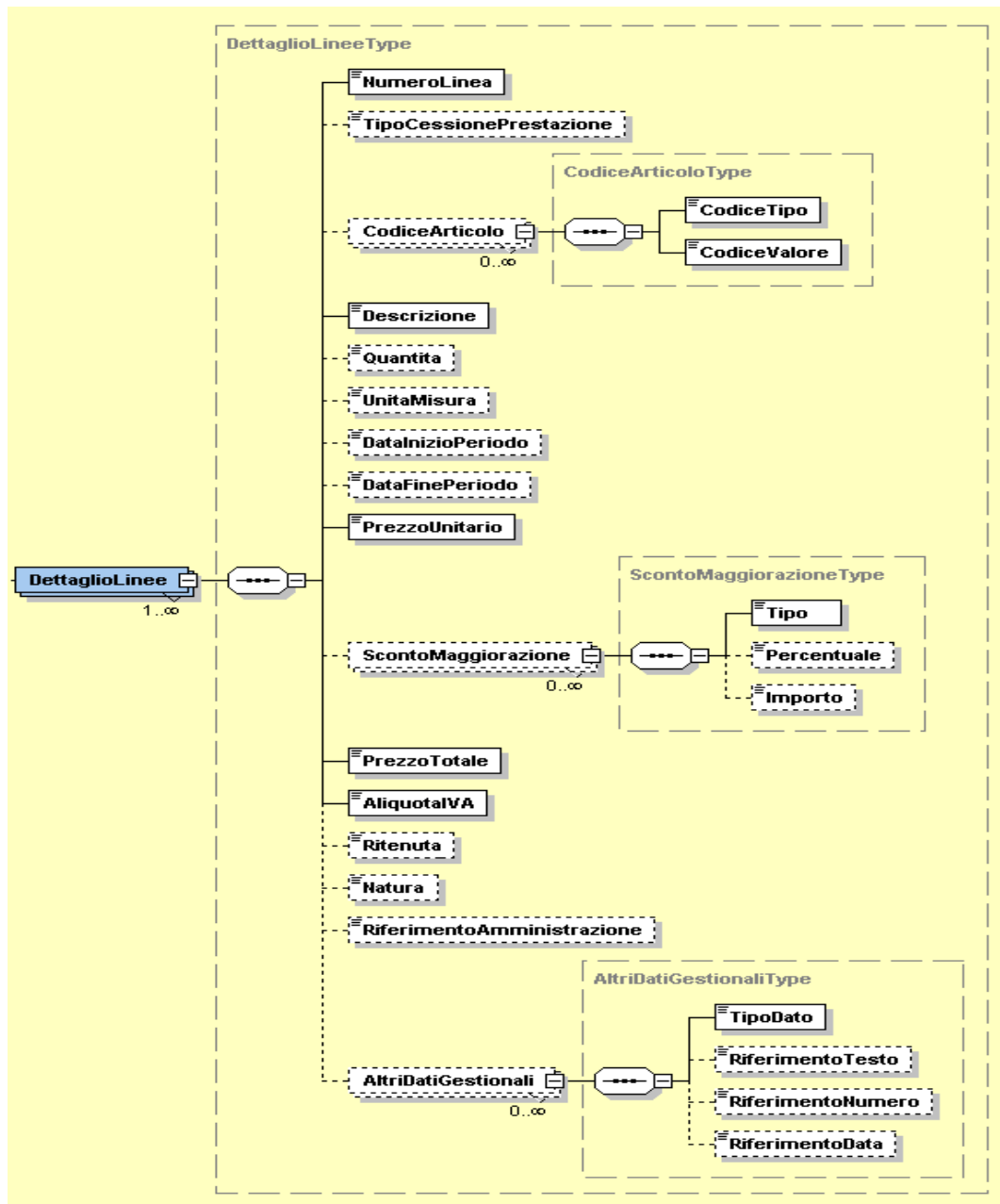
Figura 27: Elemento DettaglioLinee
