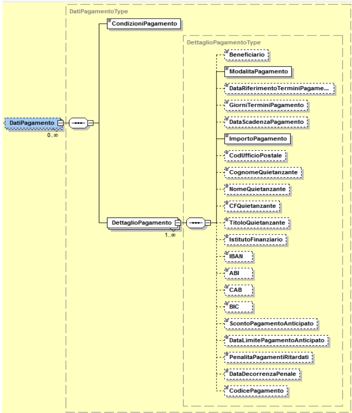
Figura 30: Elemento DatiPagamento
