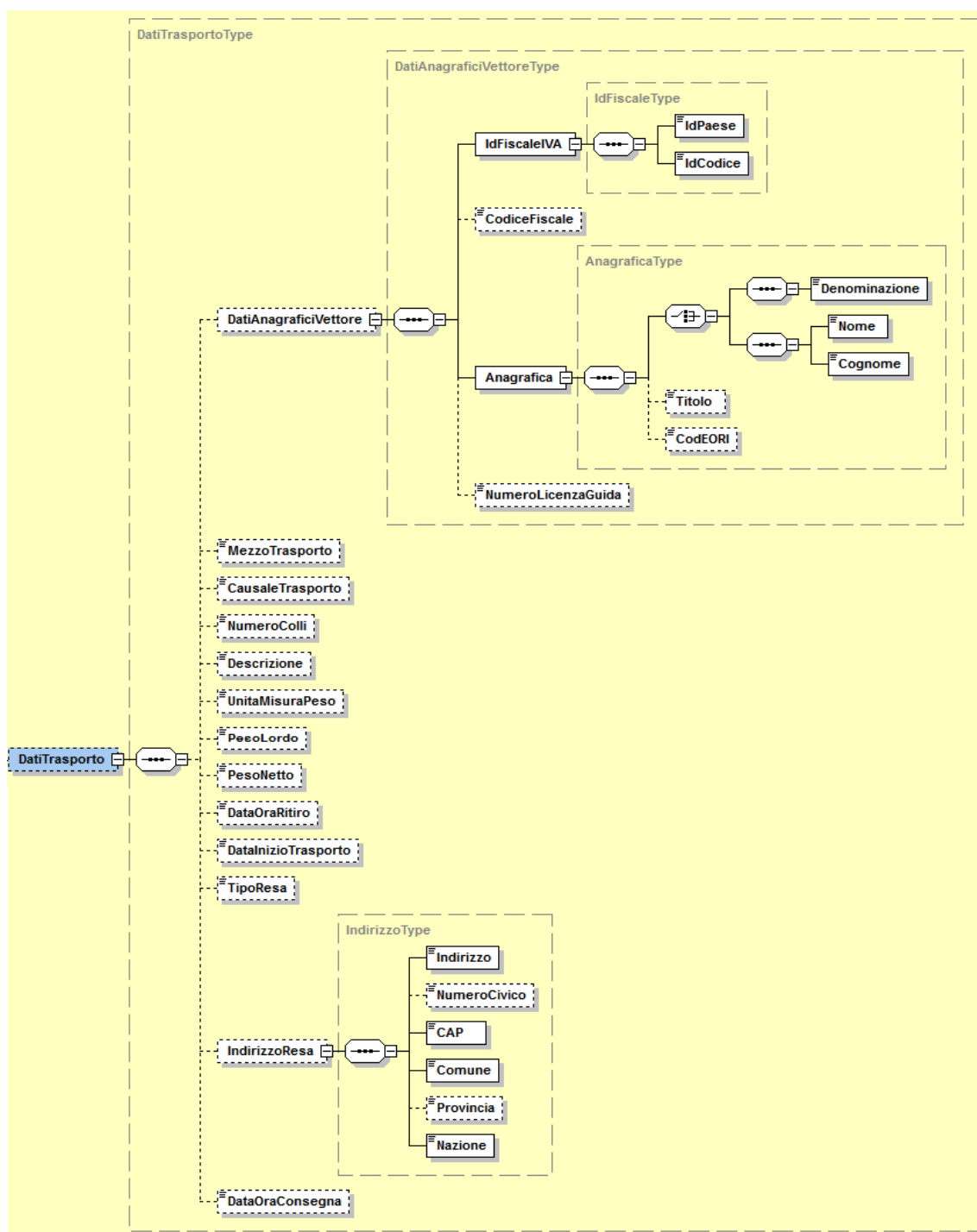
Figura 24: Elemento DatiTrasporto
