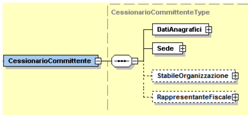
Figura 12: Elemento CessionarioCommittente
