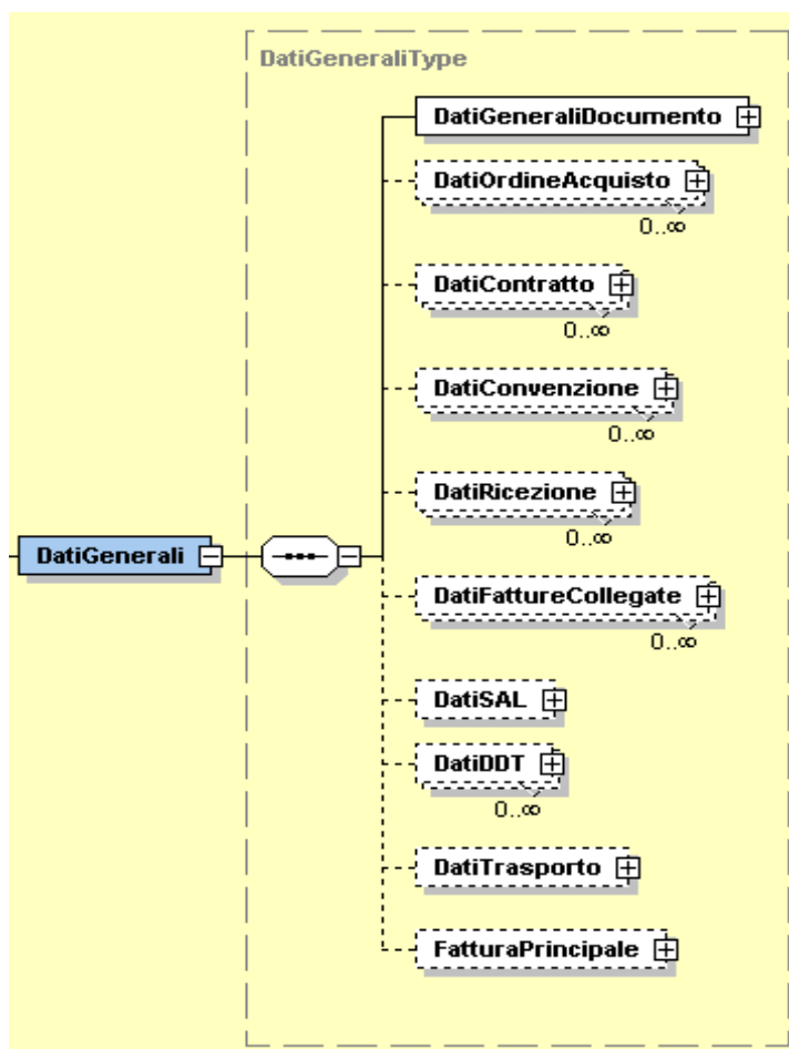
Figura 18: Elemento DatiGenerali
