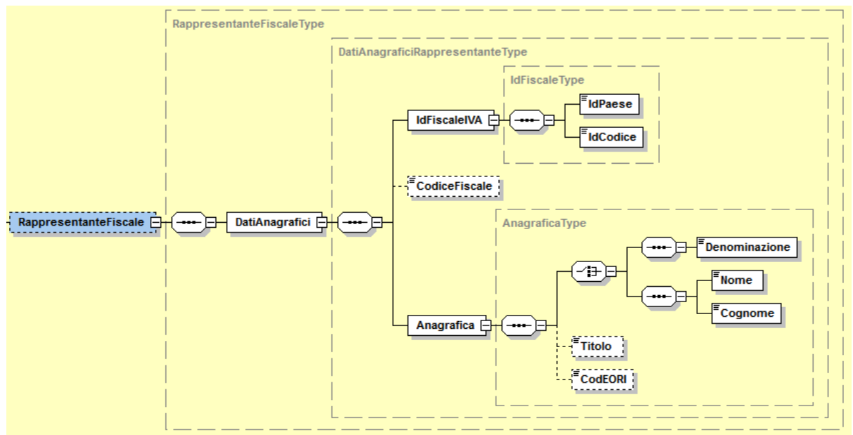
Figura 11: Elemento RappresentanteFiscale
