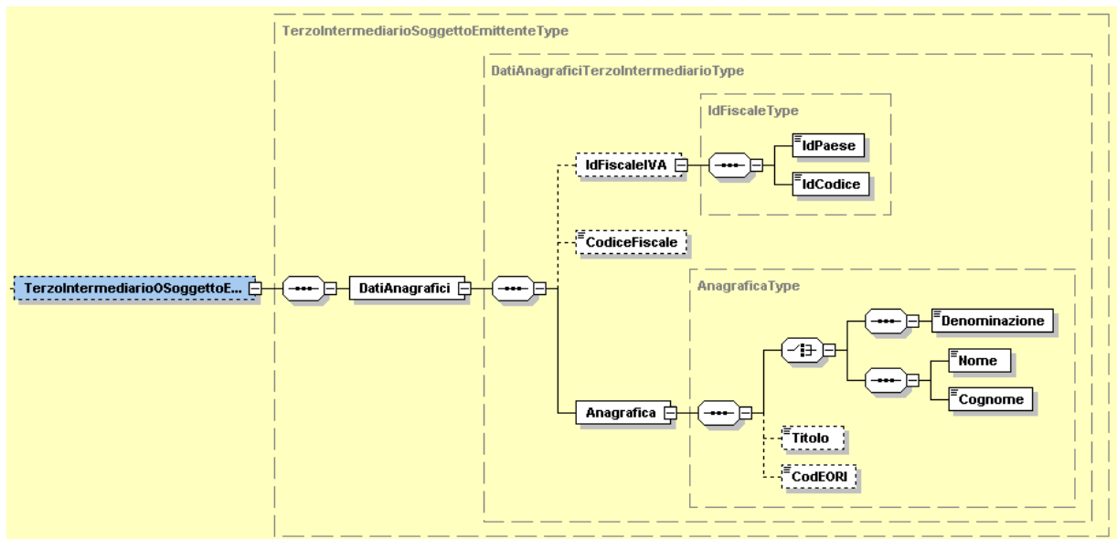
Figura 17: Elemento TerzoIntermediarioSoggettoEmittente
